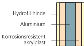
Snittegning af Korrosions hæmmende varmeveksler
